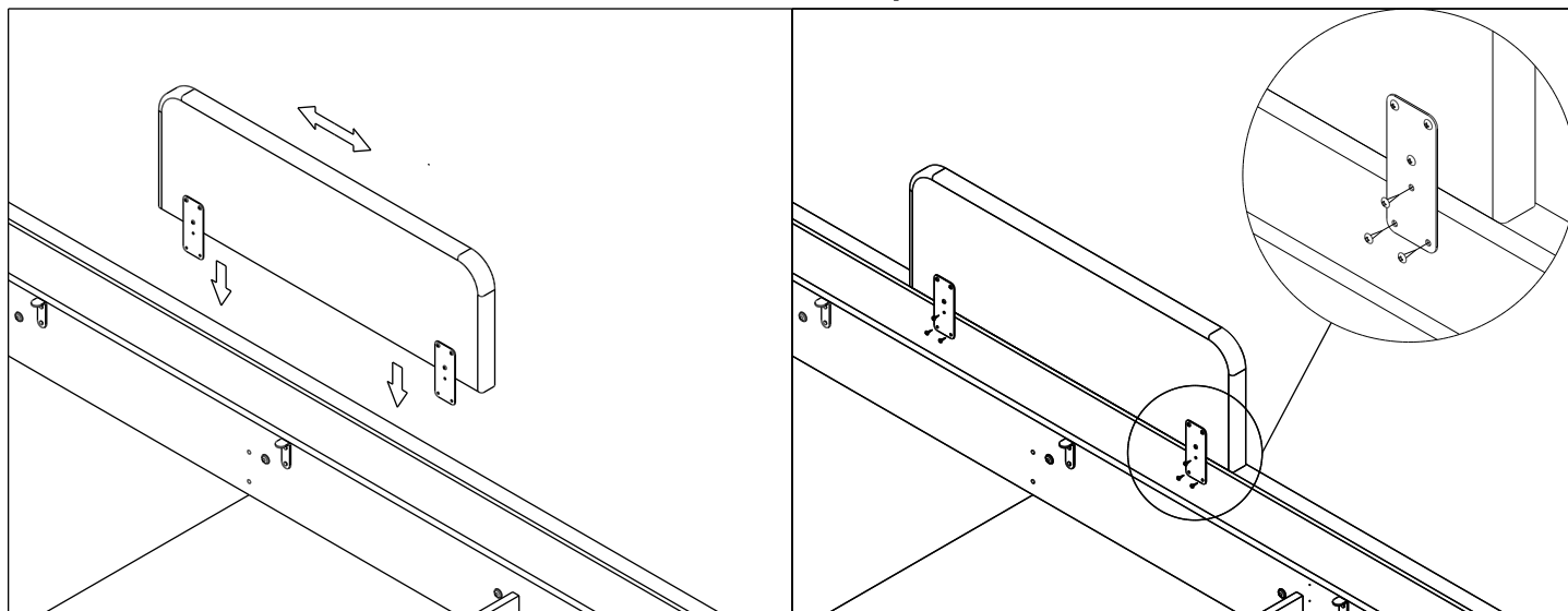
Схема 2. Установка ограничителя
