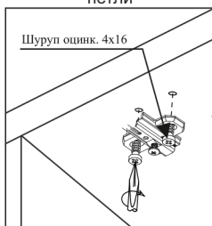
Установка ответной планки петли
