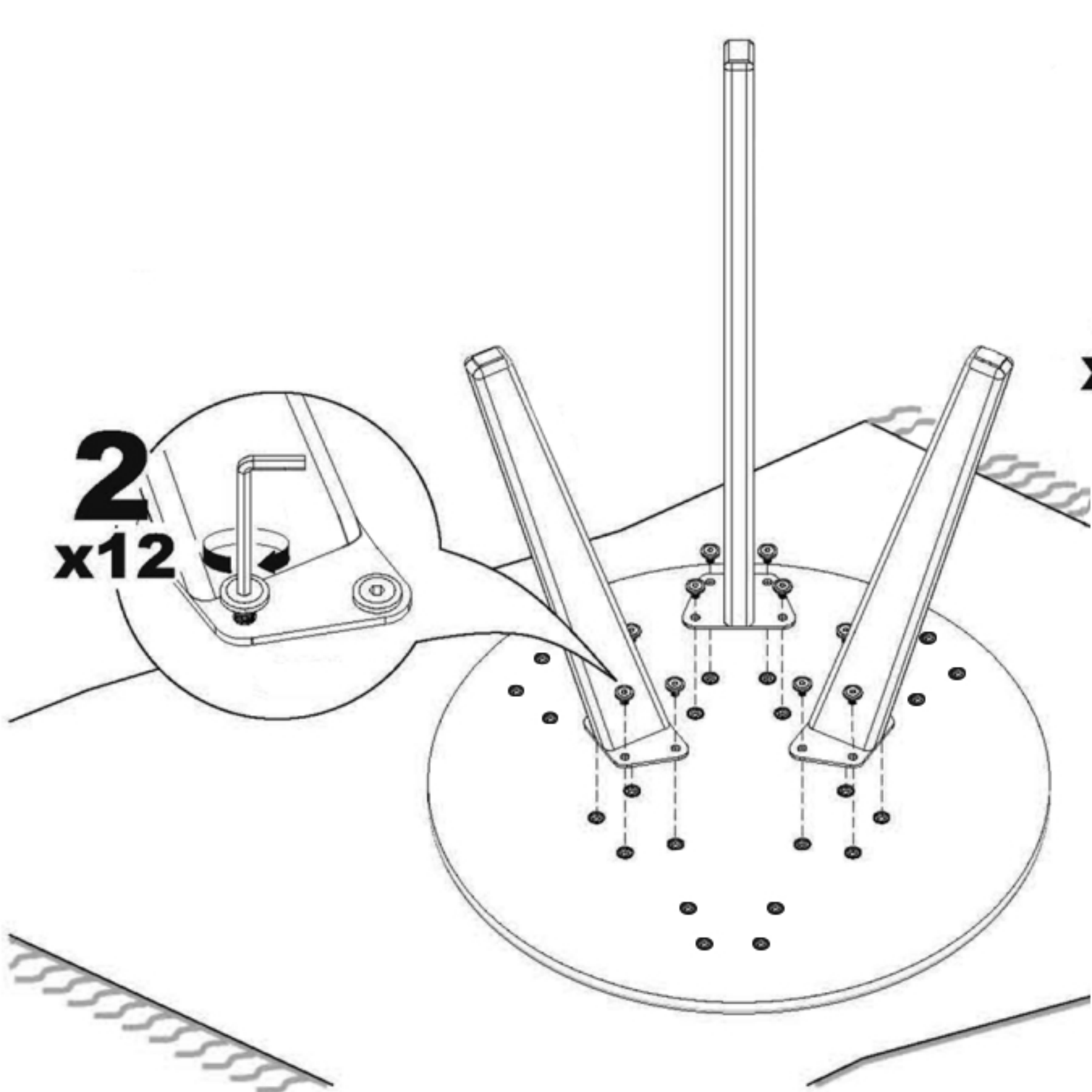
узкое крепление опор
