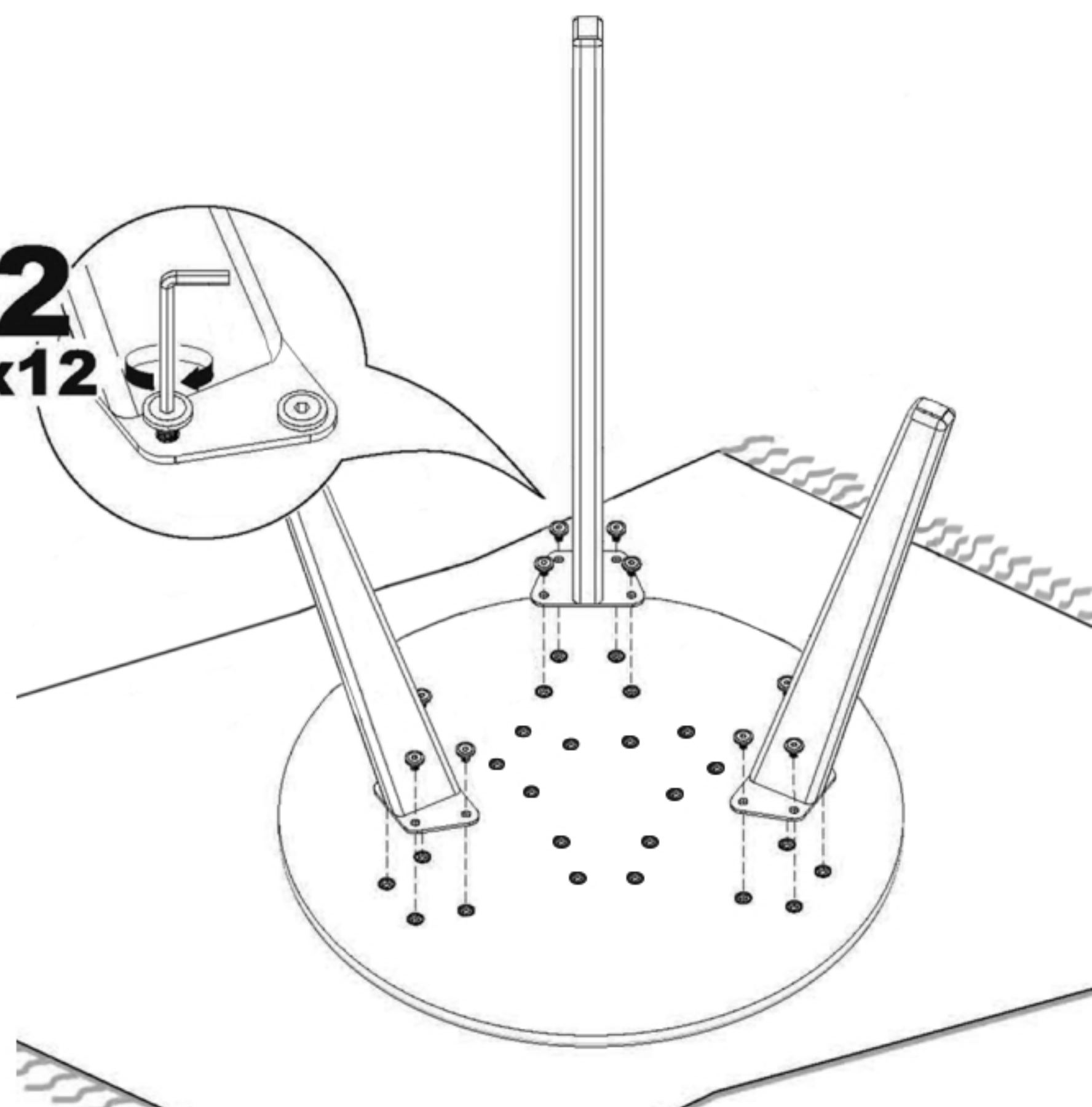
широкое крепление опор
